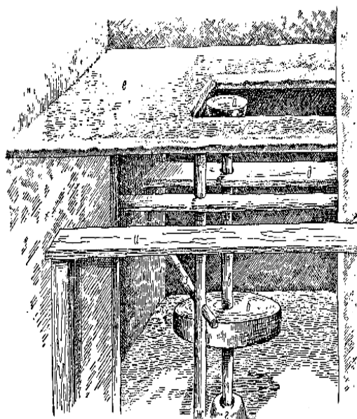
2-расм. Кулолчилик чархи ва унинг қисмлари:
